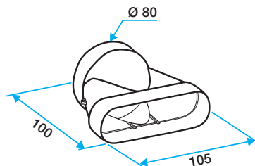
Raccord mixte pour conduit Ø80 mm
