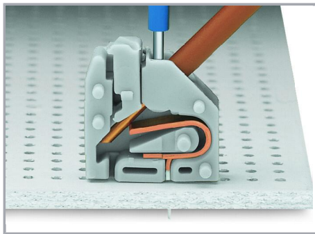
Tester avec broche de test Ø 1 mm, sur le conducteur, Série 250 – pas 2,5 mm ... 3,5 mm.
