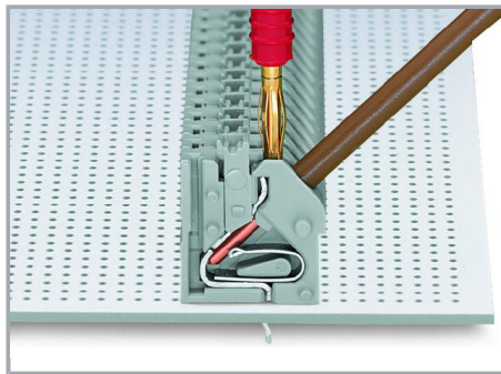
Tester avec fiche de contrôle Ø 2 mm, contact direct, Série 250 – pas 5 mm
