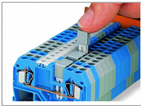
Ponter avec des contacts de pontage horizontaux (280-402) et alternants (280-409)
