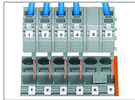
Enfichage direct des modules de fiches de contrôle dans les logements de pontage des rails conducteurs (ici série 284).
