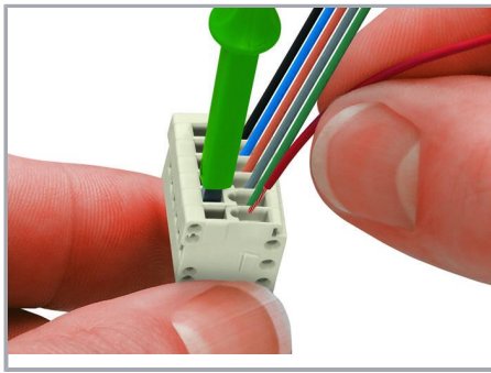
Raccordement du conducteur – avec outil de manipulation (233-335) dans l'axe du conducteur.
