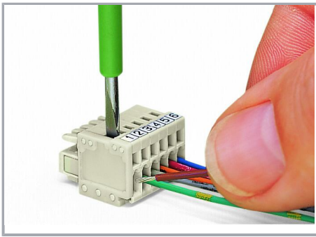
Raccordement du conducteur – avec outil de manipulation (2,5 x 0,4) mm. Perpendiculairement à l'axe du conducteur.
