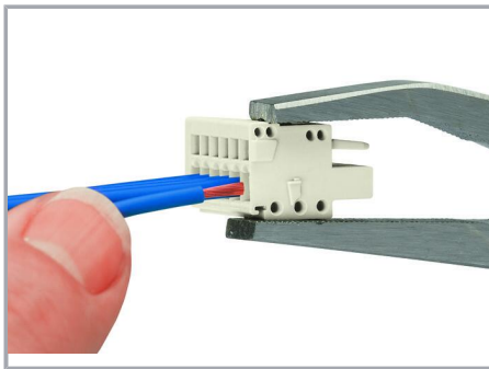
Raccordement des conducteurs avec outil de manipulation 210-251.
