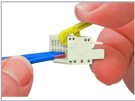
Raccordement des conducteurs avec outil de manipulation 733-191.
