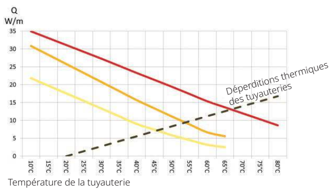
PUISSANCE DE SORTIE DES RUBANS CHAUFFANTS
