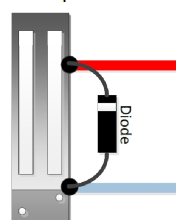
Ventouse ou gâche à rupture
