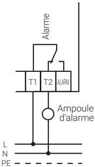
Branchement d'une ampoule (schéma) ou d'une sirène d'alarme (en repos)
