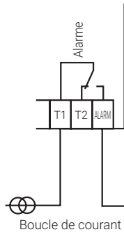
Connexion d'une boucle de courant (en repos)
