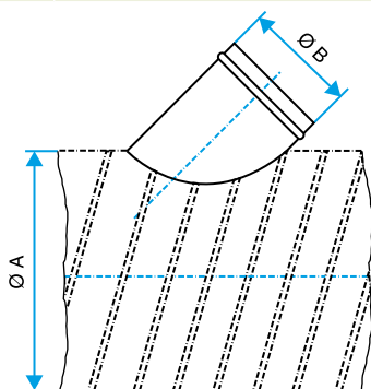
Schéma d'encadrement Piquage Oblique Circulaire 45°
