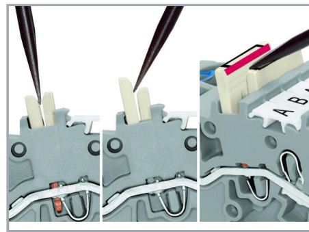
Démonter un pont intercalable.
