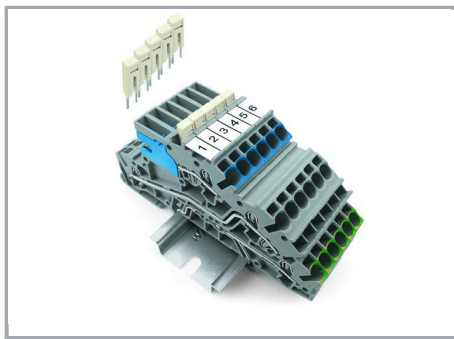
Contact de pontage horizontal pour pontage continu (2002-400)
