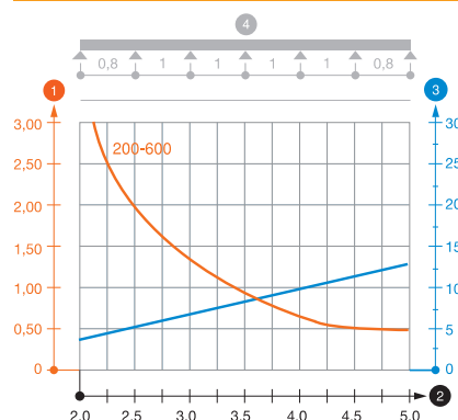
Diagramme de charge de l'échelle à câbles LG 110 VS
