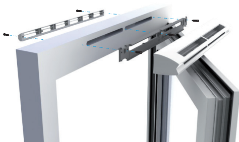
Mise en œuvre entrée d'air EHL
