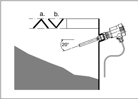
Abb. 2: Horizontaler Einbau
