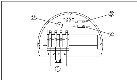
Fig. 21: Version : électronique „T“ - transistor (NPN/PNP)
