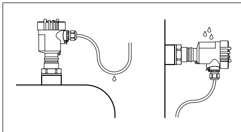
Fig. 17: Mesures prises contre l'infiltration d'humidité
