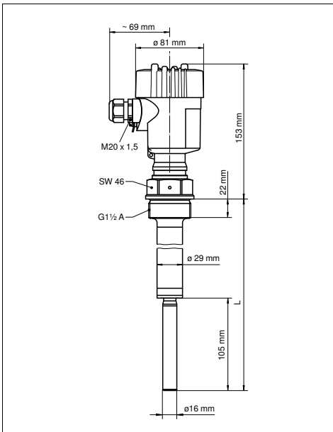
Abb. 8: Ausführung: Sensorlänge „C“, „D“ L Sensorlänge, siehe Kapitel "Technische Daten"
