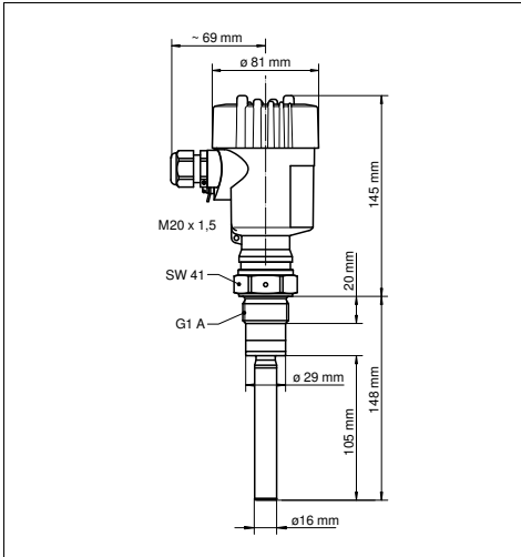
Abb. 7: Ausführung: Sensorlänge „A“
