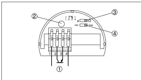
Abb. 5: Ausführung: Elektronik „T“ - Transistor (NPN/PNP)
