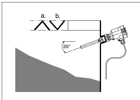
Fig. 26: Montaje horizontal
