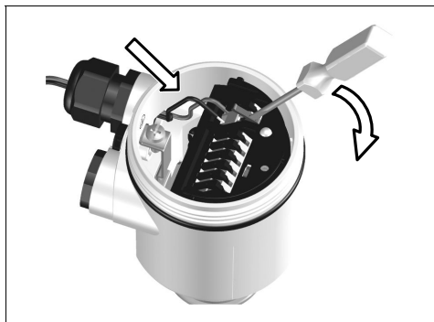
Abb. 3: Anschlusschritte 5 und 6
