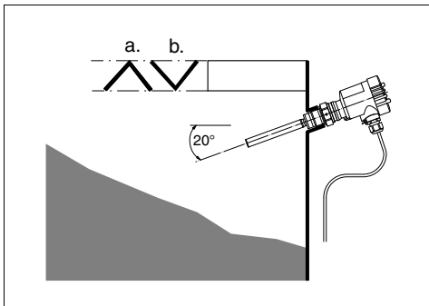
Fig. 18: Montage horizontal
