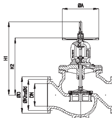
MSV-F2 DN 200 - 400
