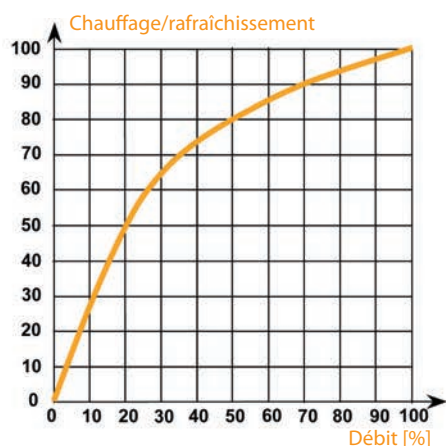
Echangeur de CTA
