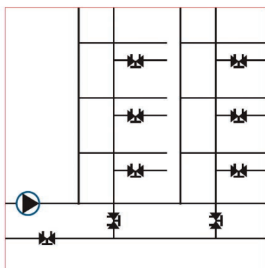
Équilibrage avec vannes manuelles.
