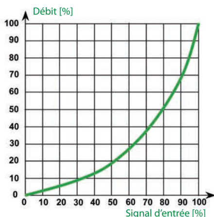
AB-QM + AME 435 QM avec réglage sur logarithmique
