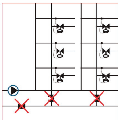
Équilibrage avec vannes automatiques.
