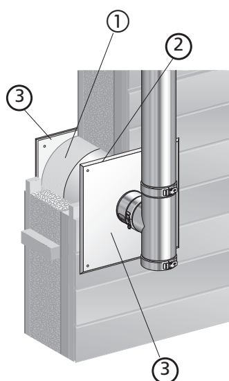
① COQISOL ② PDSE ③ PPI (x2)
