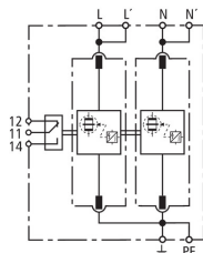
Schéma de principe du circuit DV M TN 255 FM
