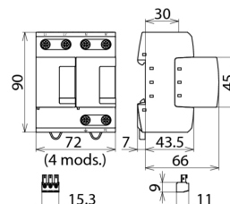
Dimensions DV M TT 255
