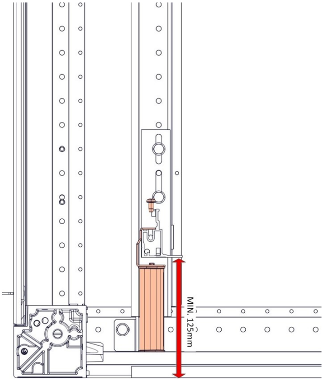
Vue de dessus — Top view
