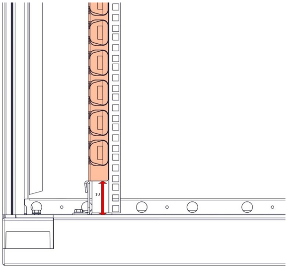
Vue de face — Front view
