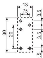
95.13.2 Vue côté cuivre
