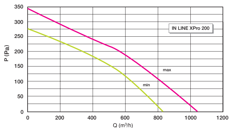
Courbe aéraulique XPro 200
