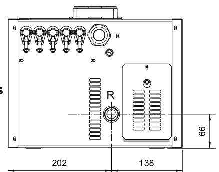
Vue dessous
