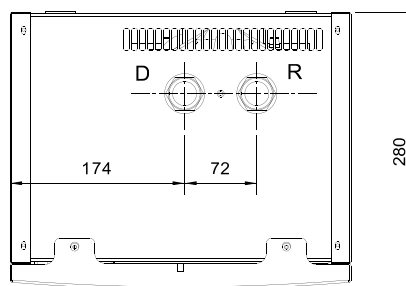
Vue dessus
