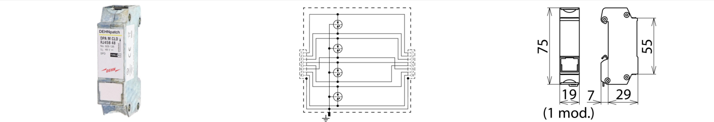
Illustrations sans engagement Schéma de principe du circuit DPA M CLD RJ45B 48 Dimensions DPA M CLD RJ45B 48
