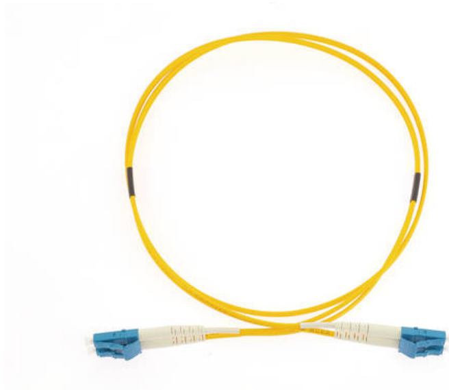
Jarreti res optiques duplex OS2 9/125  m, gaine jaune.
