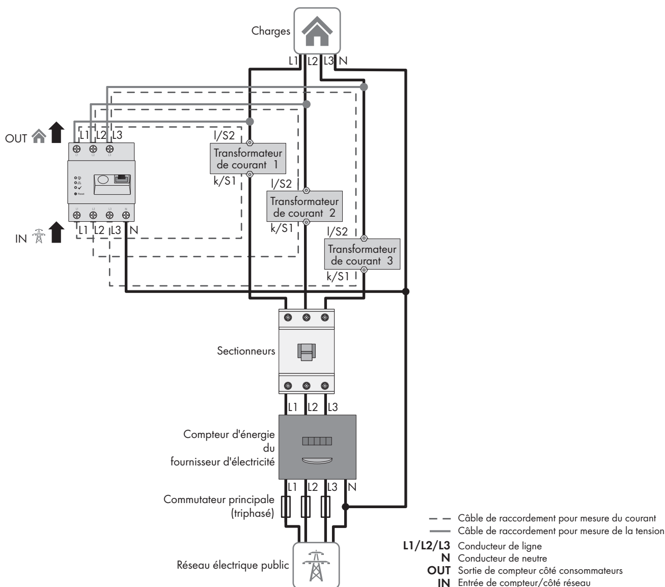
Figure 6 : Exemple de connexion dans des schémas TN et TT, en cas d'installation sur le point de raccordement au réseau
