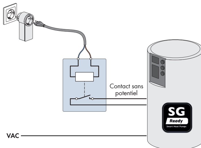
Figure 21 : Raccordement d'une pompe à chaleur via une prise radiocommandée compatible et un relais séparé
