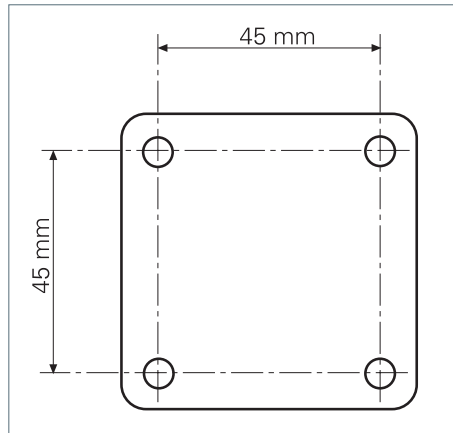
Fig. 2: Bohrbild.
