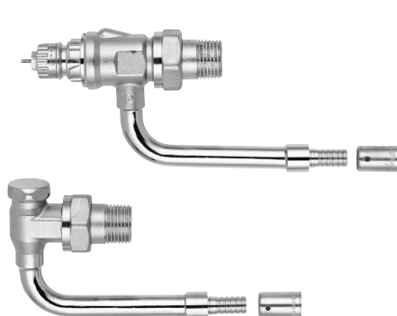
RA-N/HC et RLV-S/HC, à sertir
