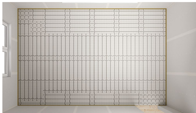
*schéma d'installation avec deux boucles de chauffage
