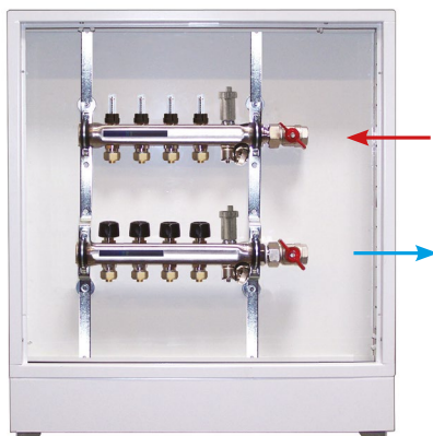
Alimentation horizontale (coffrets encastrés ou apparents)
