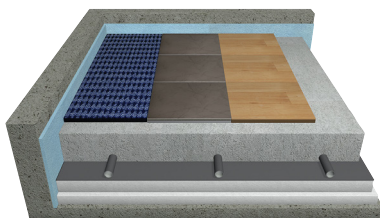
Constitution de plancher chauffant traditionnel
