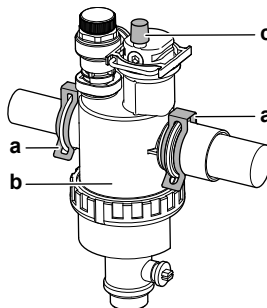
a Fermoir b Filtre magnétique/pot de décantation c Vanne de purge d'air
