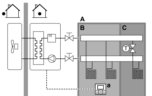
A Zone de température de départ principale B Pièce 1 C Pièce 2 a Interface utilisateur utilisée en tant que thermostat d'ambiance
