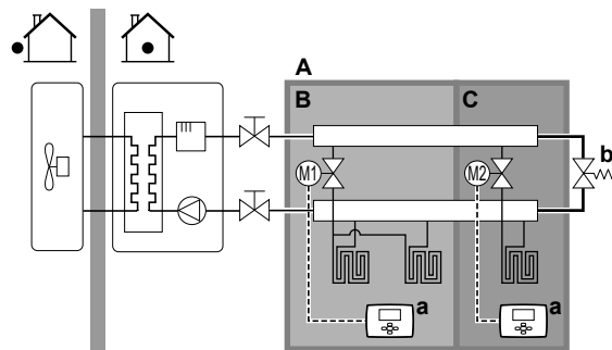
A Zone de température de départ principale B Pièce 1 C Pièce 2 a Thermostat d'ambiance externe b Vanne de dérivation
