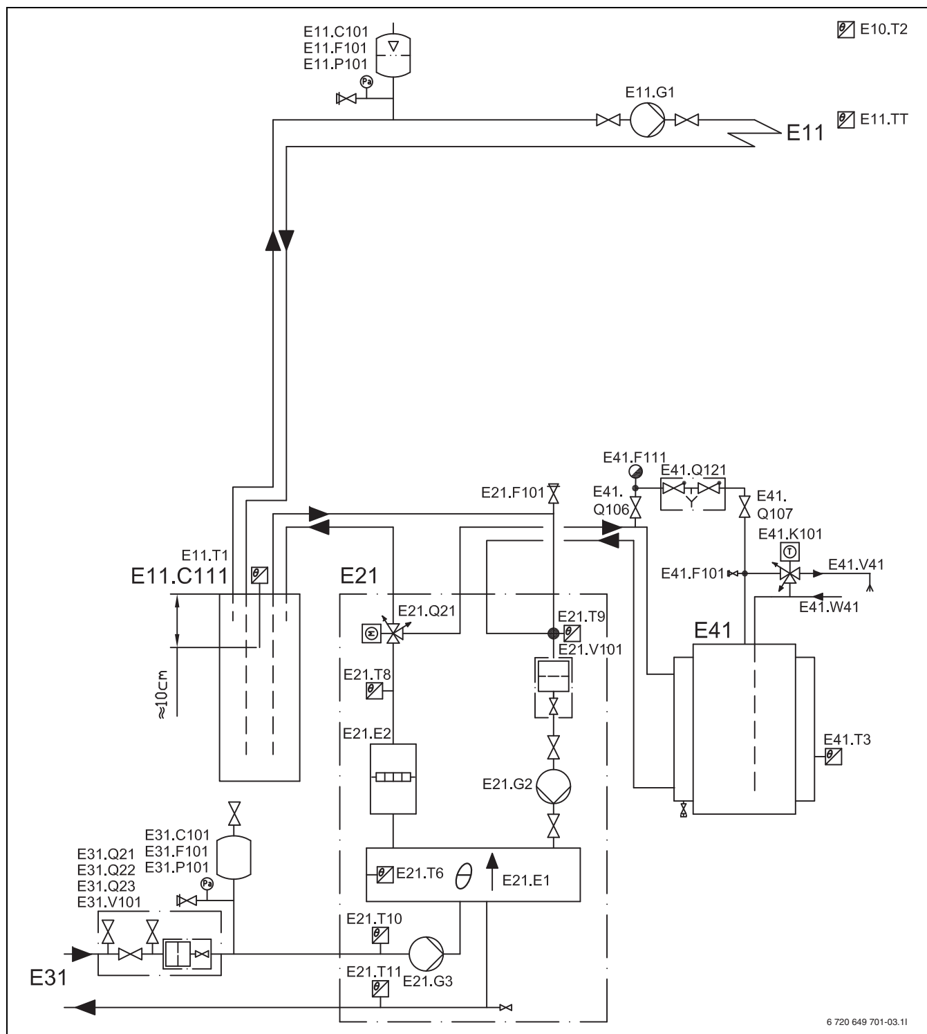
Fig. 13 Circuit de chauffage sans vanne mélangeuse avec réservoir de service et ballon d'eau chaude extérieure
