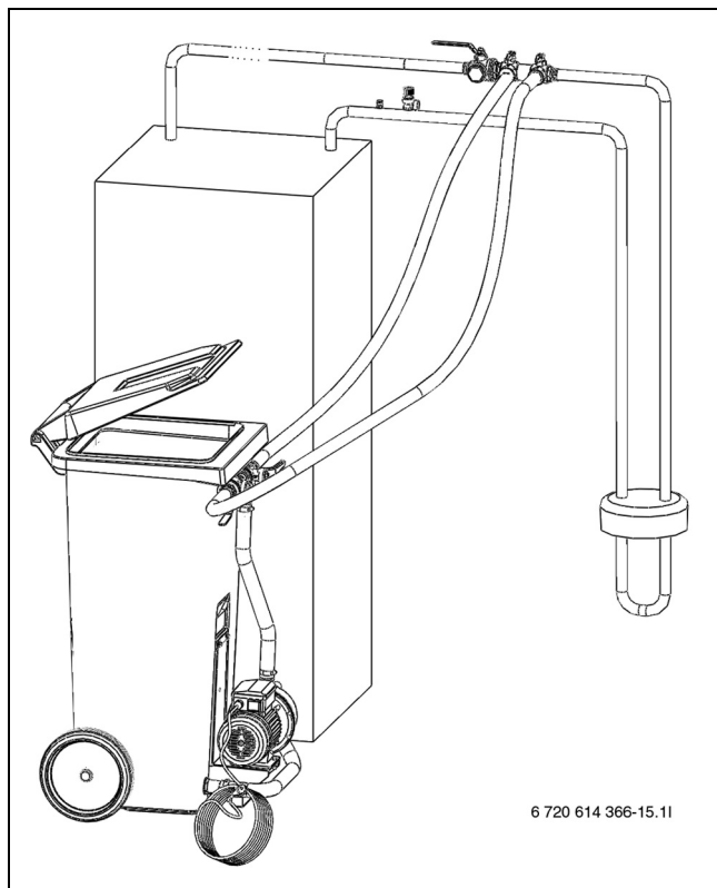
Fig. 21 Remplissage avec station de remplissage
