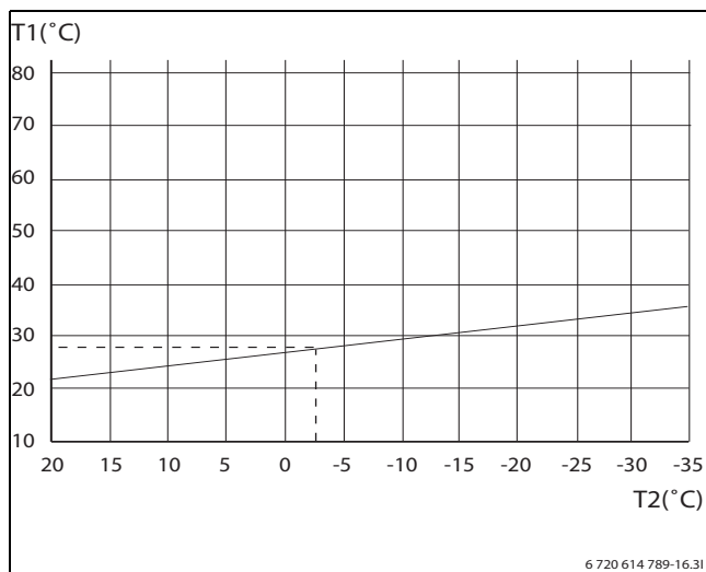
Fig. 43 Plancher
