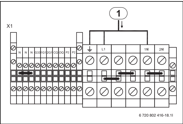
Fig. 30 Alimentation électrique
