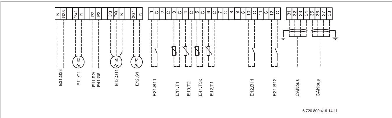
Fig. 34 Connexions externes
