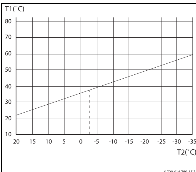
Fig. 42 Radiateur
