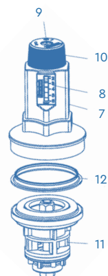
Fig. 4 - Unità funzionale ridotta di pressione solo per E1 NEU HWS
