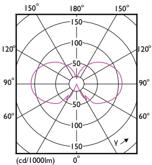
LEDbulb CLA A67 11,5W E27 827 FR
