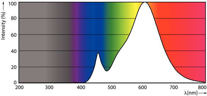
LEDbulb CLA 11,5W A67 E27 827 FR
