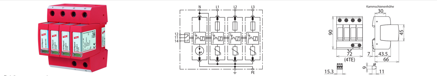
Schéma de principe du circuit DG M TT 5 CI 275 NL FM Dimensions DG M TT 5 CI 275 NL FM
