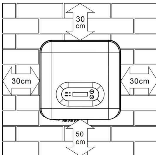
Figure 10 – Distance pour un seul onduleur
