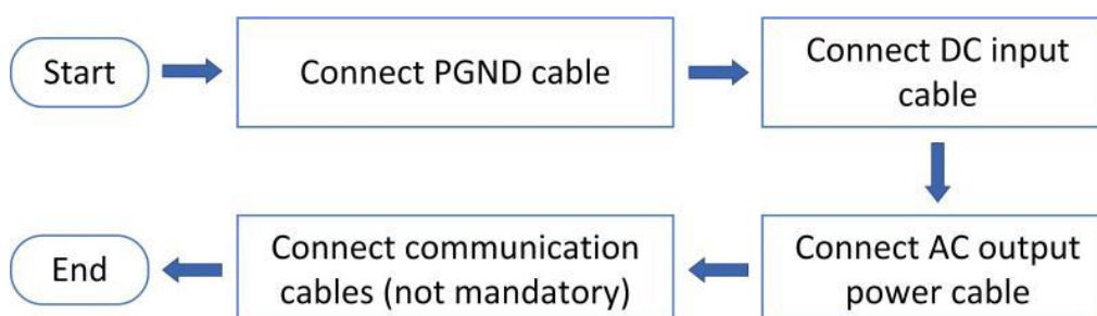
Figure 8 – Phases pour la connexion des câbles
