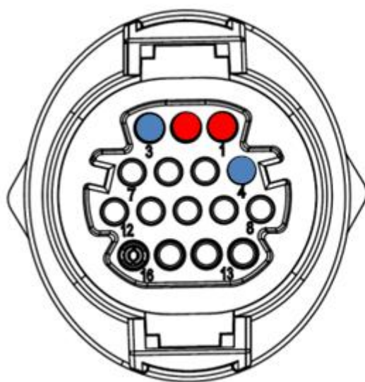
Figure 82 – Connexion ligne série via connecteur de communication pour 3PH HYD5000-HYD20000-ZSS
