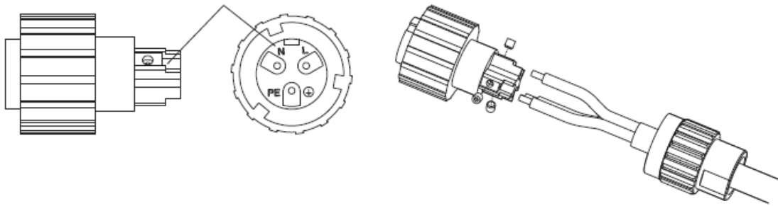
Figure 20 – Connexion des câbles de sortie AC (3)
