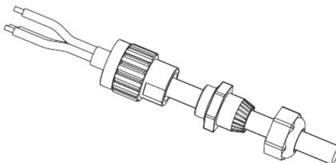
Figure 19 – Connexion des câbles de sortie AC (2)
