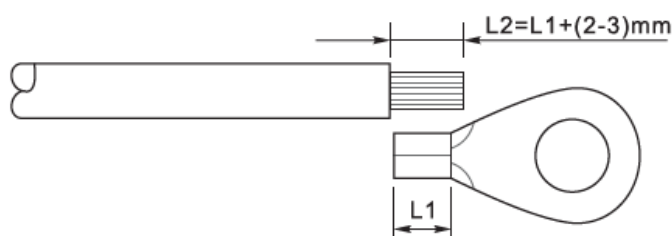
Figure 9 – Préparation du câble de terre (1)
