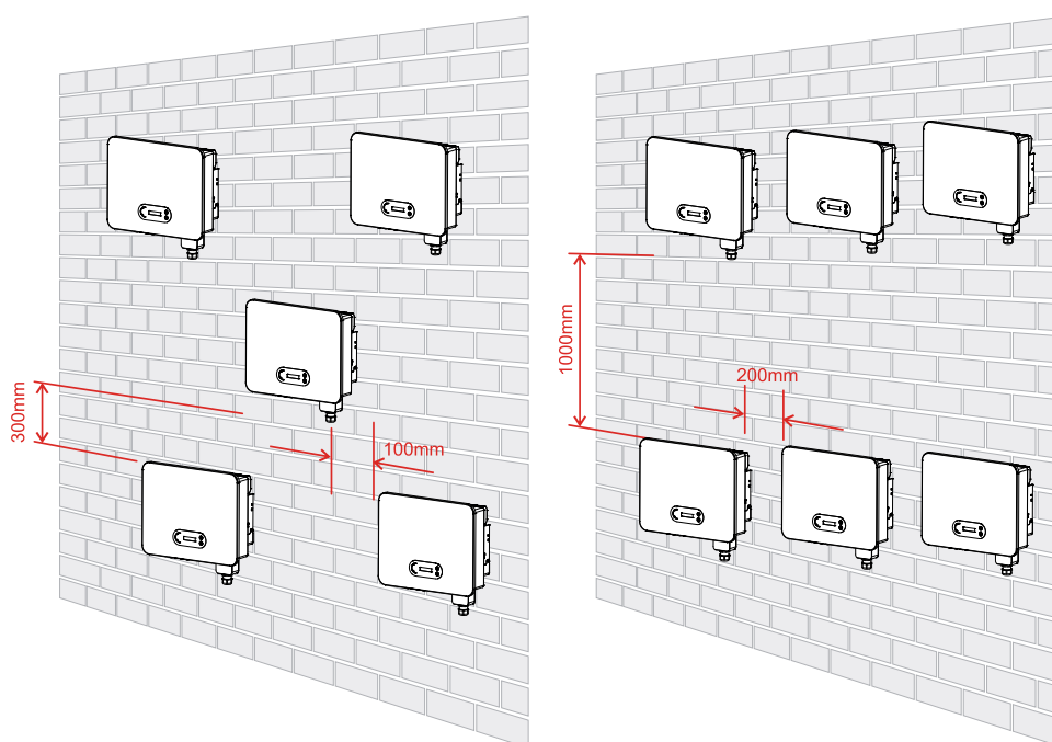
Figure 11 – Distance pour plusieurs onduleurs
