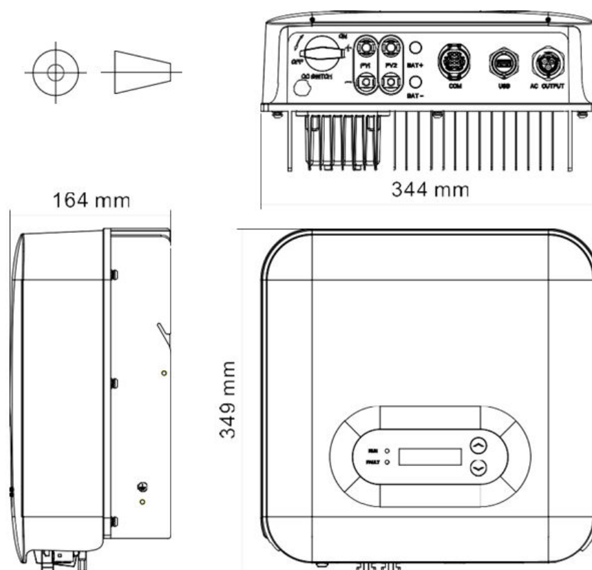
Figure 3 – Vues de face et latérale de l'onduleur
