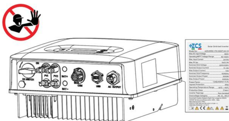
Figure 5 – Ne pas enlever l'étiquette sur le côté de l'onduleur
