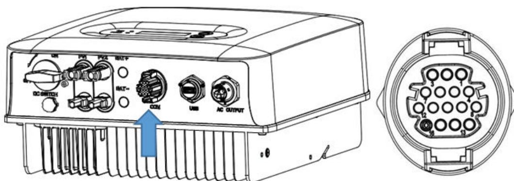
Figure 23 – Vue de dessous de l'onduleur 1PH 3000TLM-6000TLM-V3
