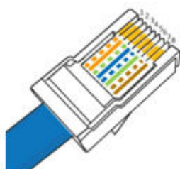
Figure 78 – Broches en sortie pour la connexion du connecteur RJ45
