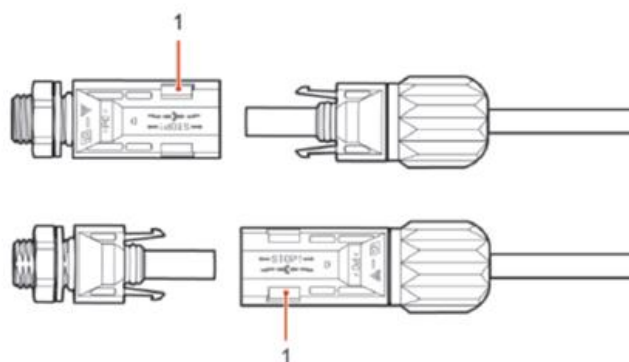
Figure 15 – Raccordement des câbles d'alimentation en entrée DC (3)
