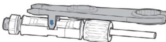
Figure 16 – Retrait du connecteur DC
