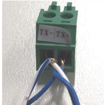
Figure 80 – Serrage du câble de réseau au bornier RS485
