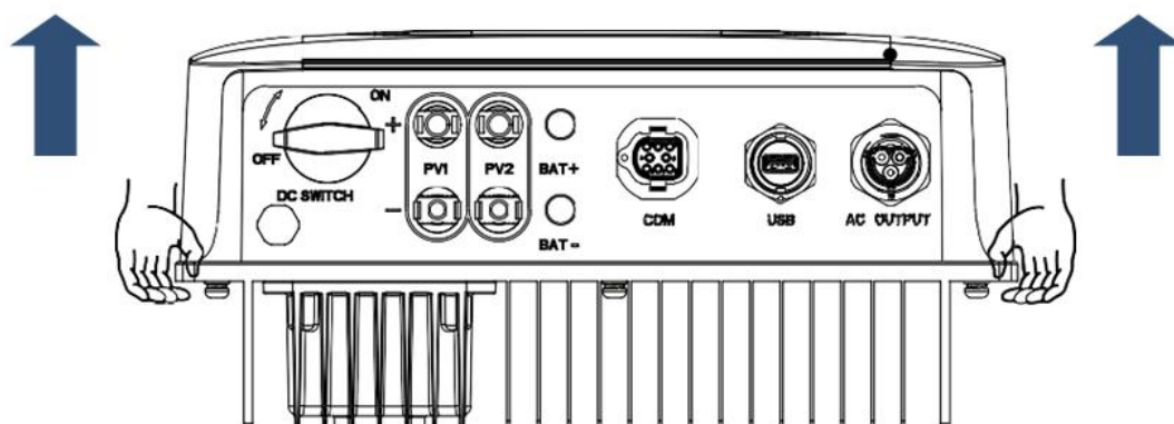
Figure 6 – Extraction de l'onduleur de l'emballage
