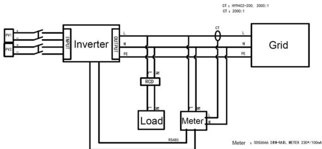
Figure 26 – Schéma B : Compteur +CT
