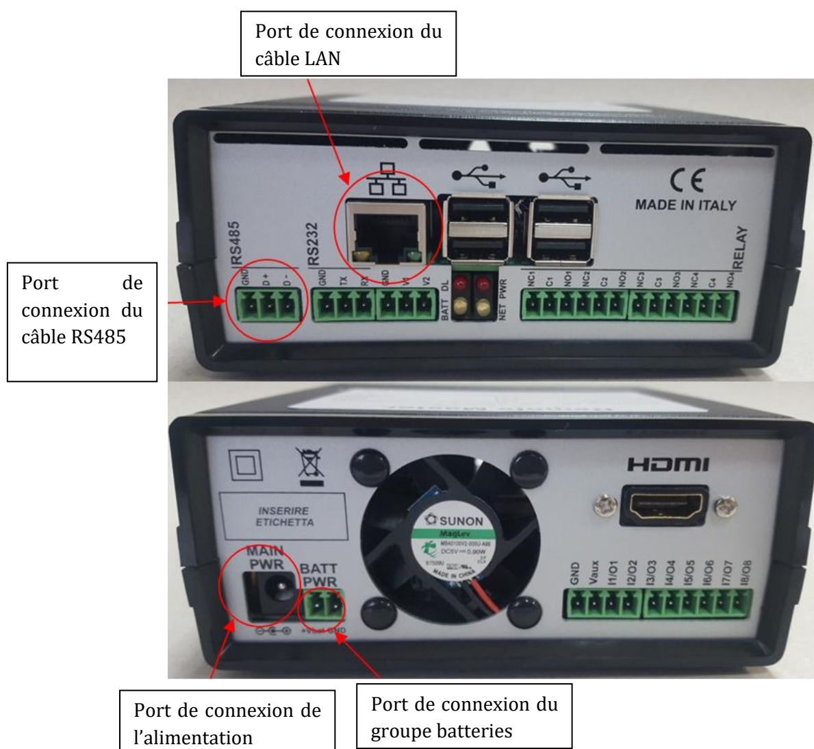
Figure 102 : Panneau arrière du datalogger
