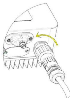
Figure 22 – Déconnexion des câbles de sortie AC
