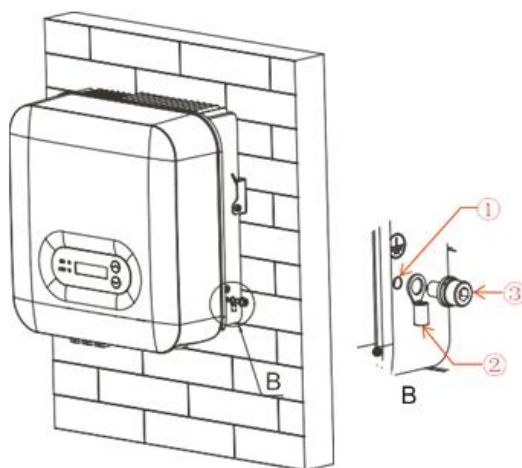
Figure 18 – Diagramme des instructions de mise à la terre à l'extérieur de l'onduleur
