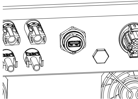
Figure 39 – Retrait du capot de la carte de communication
