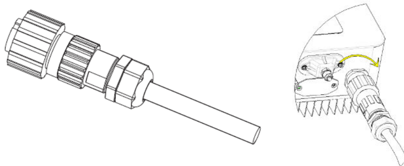
Figure 21 – Connexion des câbles de sortie AC (4)
