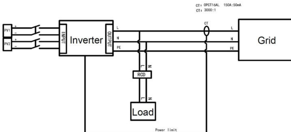
Figure 25 – Schéma A : CT (prédéfini)
