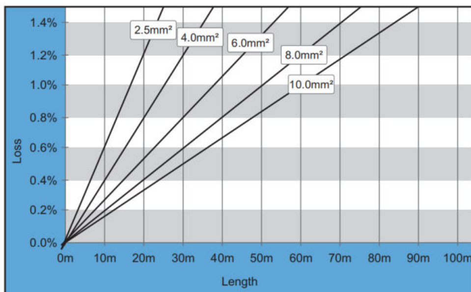
Figure 26 – Rapport entre longueur du câble, aire de la section transversale et puissance dissipée
