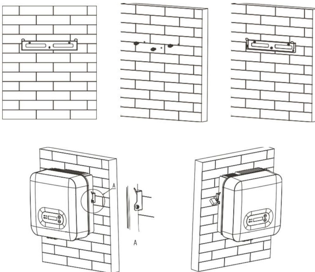
Figure 7 – Phases pour le montage de l'onduleur au mur
