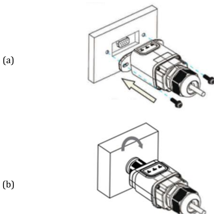
Figure 64 – Introduction et fixation de l'adaptateur Ethernet
