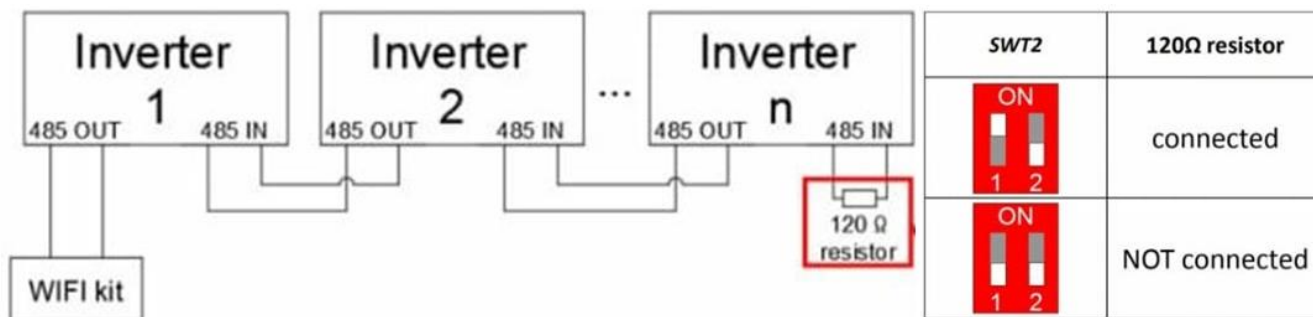
Figure 83 – Position des commutateurs DIP pour connecter la résistance d'isolement
