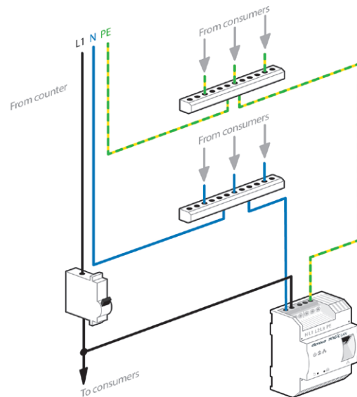
Β) 1-φασική εγκατάσταση χωρίς αυτόματο διακόπτη διαρροής
