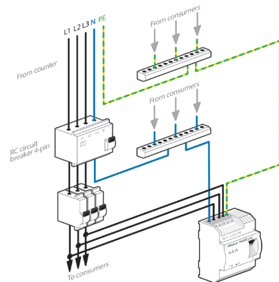
Γ) 3-φασική εγκατάσταση με αυτόματο διακόπτη διαρροής
