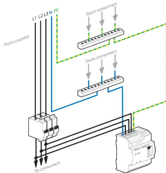
A) 3-φασική εγκατάσταση χωρίς αυτόματο διακόπτη διαρροής
