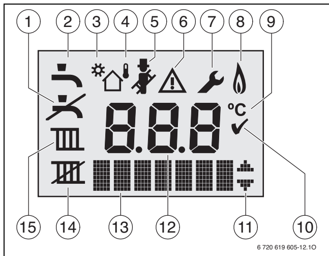
Fig. 6 Messages d'écran
