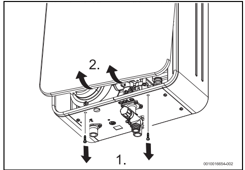
Fig. 25 Retirer l'habillage avant.
