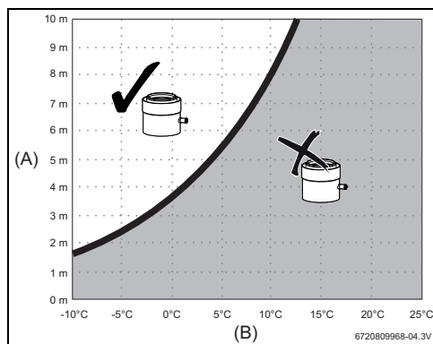
Fig. 22 Tuyaux concentriques
