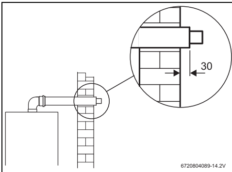
Fig. 20 Dimensions (en mm)
