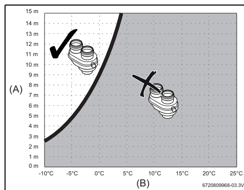
Fig. 23 Tuyaux séparés
