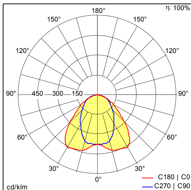
D41246_TECTON_C_LED16000_830_L2000_VWB_LDE_WH.Idt
