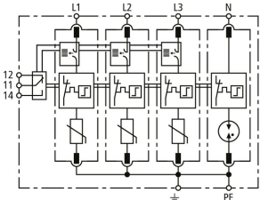
Schéma de principe du circuit DG M TNS ACI 275 FM
