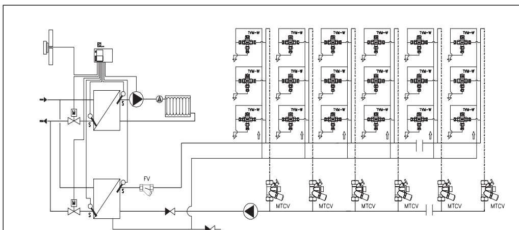
Fig. 8 : schéma d'une installation d'eau chaude avec circulation (version automotrice).
