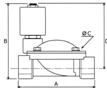
Encombrements (mm)
