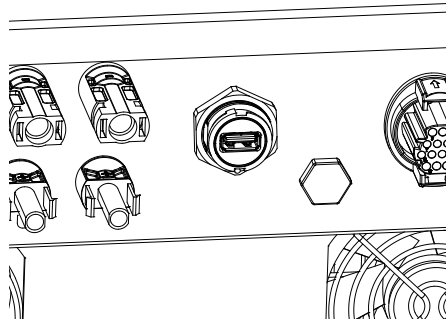
Figure 39 – Retrait du capot de la carte de communication
