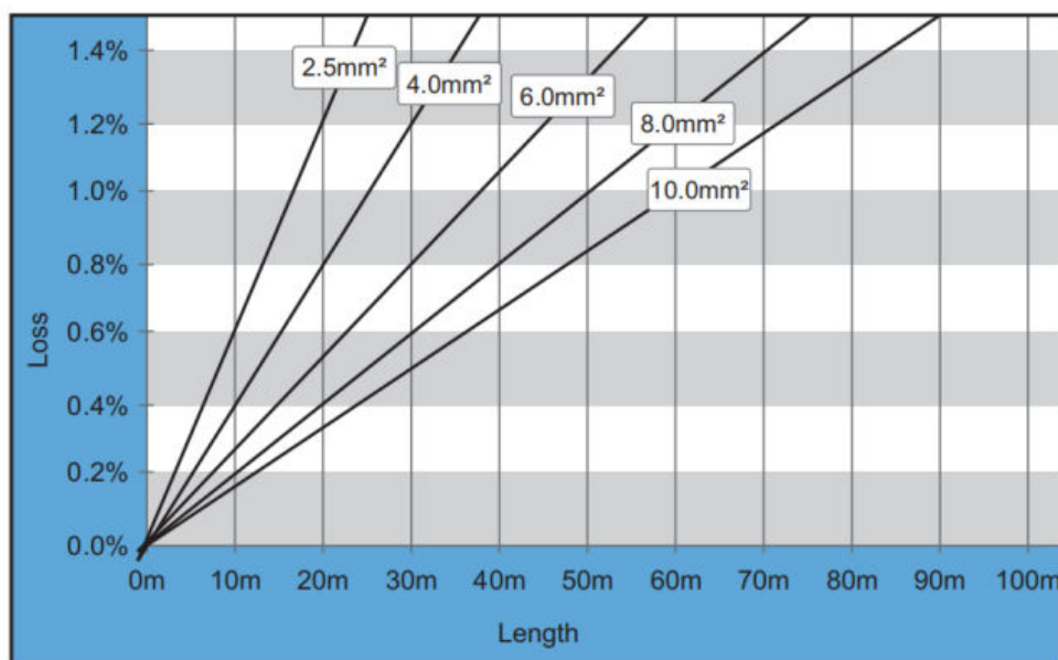
Figure 26 – Rapport entre longueur du câble, aire de la section transversale et puissance dissipée
