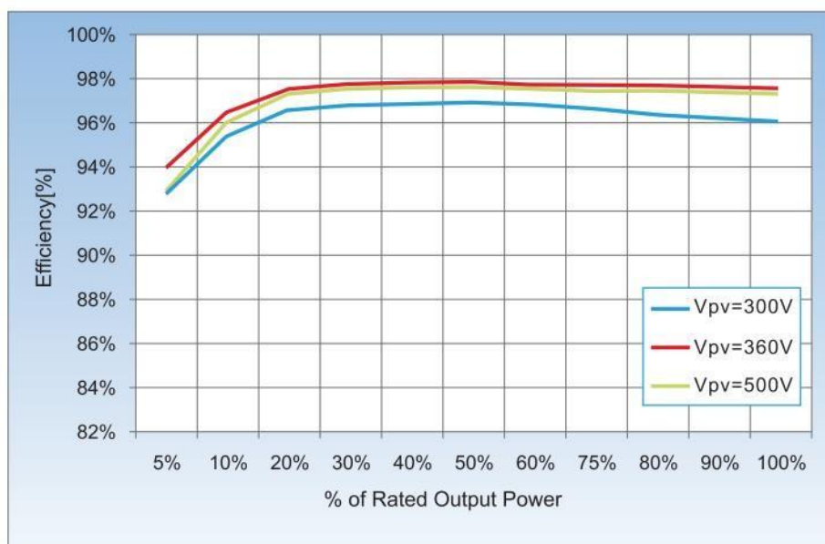
Figure 7 – Courbe de rendement énergétique
