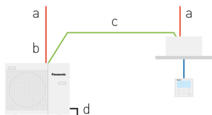
PACi PZ2/PZH2 : méthode à 2 fils
