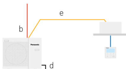
Gamme PACi NX : méthode à 3 fils
