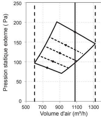
175Pa Volume d'air standard : 1080 m³/h
