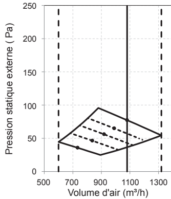
75Pa Volume d'air standard : 1080 m³/h
