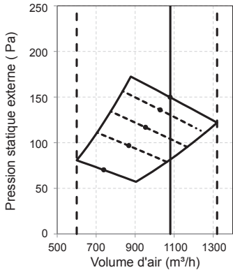
150Pa Volume d'air standard : 1080 m³/h
