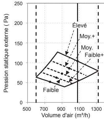
100Pa Volume d'air standard : 1080 m³/h
