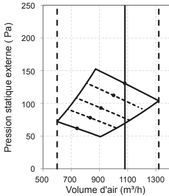
125Pa Volume d'air standard : 1080 m³/h
