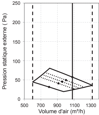
50Pa Volume d'air standard : 1080 m³/h
