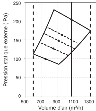
200Pa Volume d'air standard : 1080 m³/h
