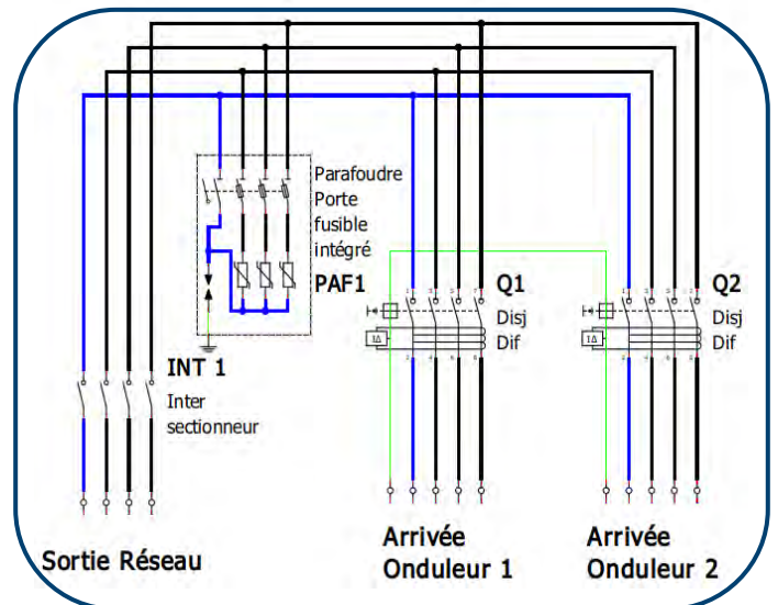
Figure 39 : Schéma de principe coffret AC TRI 2 onduleurs
