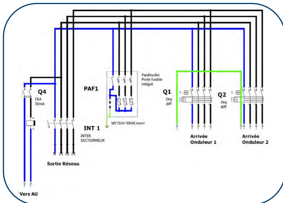
Figure 41 : Schéma de principe coffret AC TRI 2 onduleurs &lt; 36 kW
