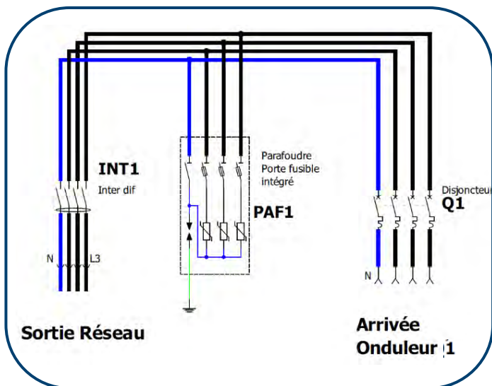
Figure 38 : Schéma de principe coffret AC TRI 1 onduleur
