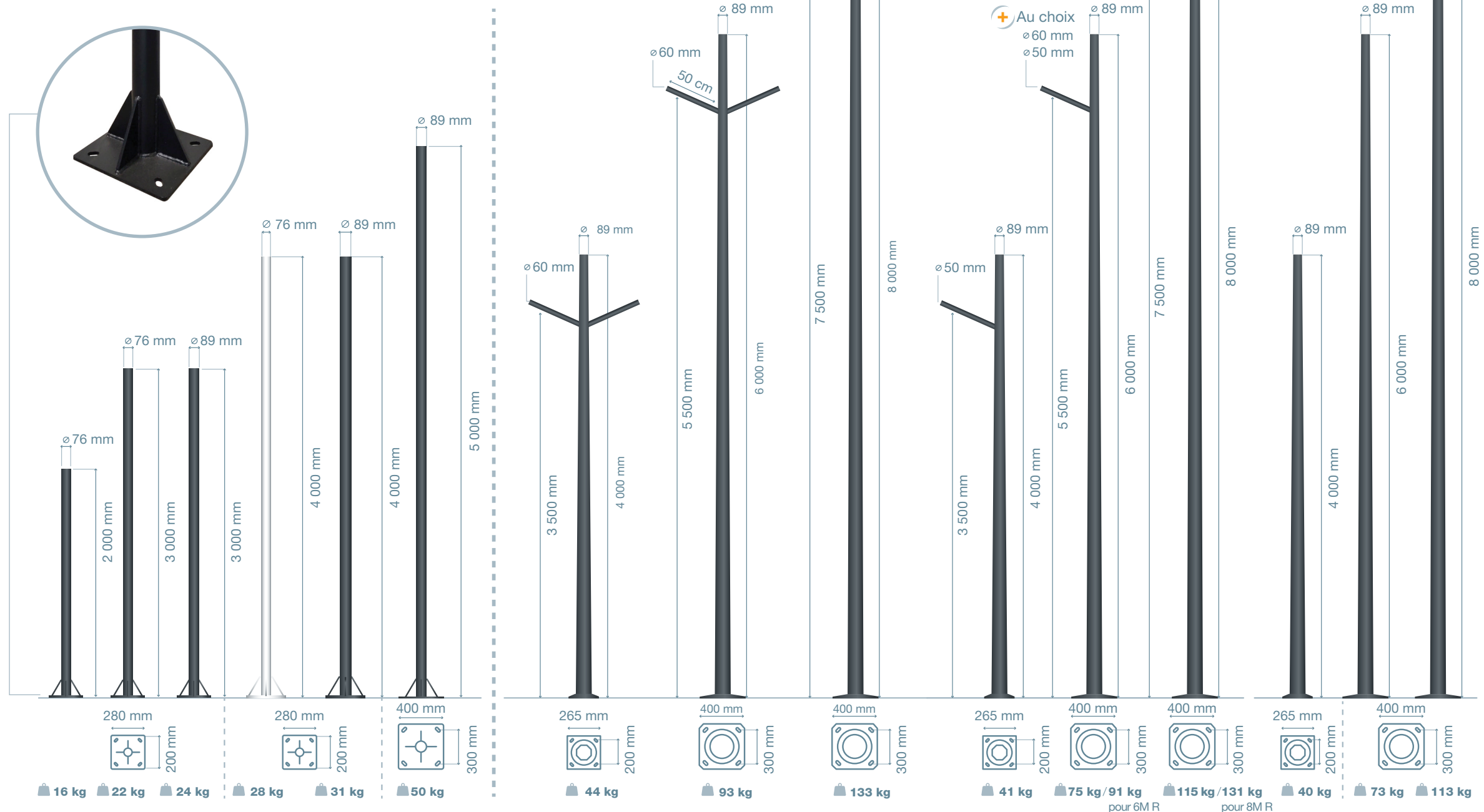
MÂTS CYLINDRIQUES
