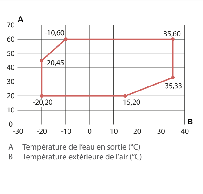
Limites de fonctionnement en chauffage
