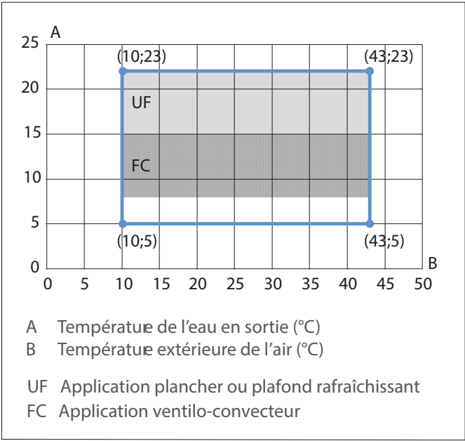
Limites de fonctionnement en refroidissement
