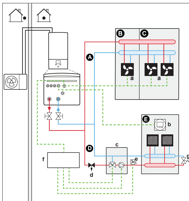
2 Système avec séparateur hydraulique pour zone principale:
