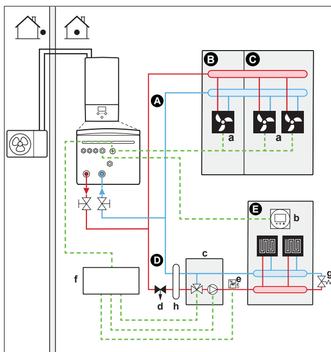
3 Système avec séparateur hydraulique pour les deux zones: Pour ce système, une pompe directe est requise pour la zone supplémentaire.
