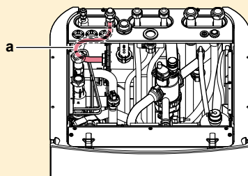
a Tuyau de gaz réfrigérant
