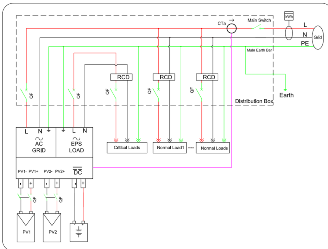
Figure 6 – Raccordements électriques
