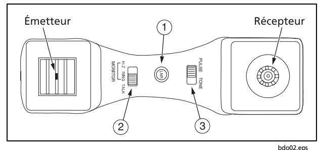
Figure 2. Commandes sur poignée
